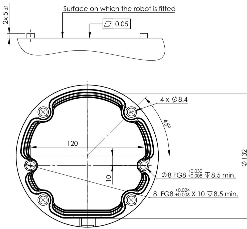
Габариты робота для монтажа и схема расположения отверстий на нем.
